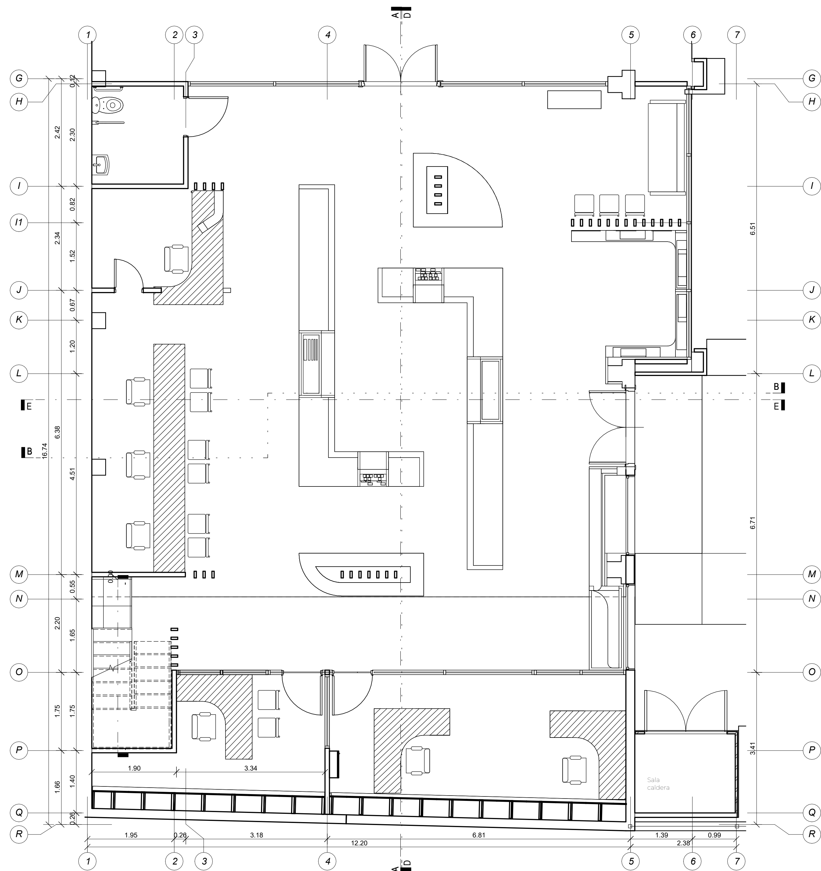
PLANTA NIVEL 1
